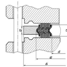
СНП-Г "с кольцевой канавкой под металлокерамическую прокладку"
